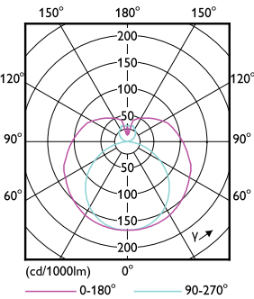
30W FA8 840 4000K
